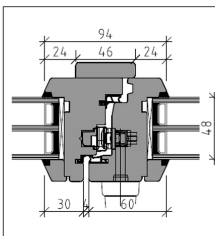
Schnitt Mittelpartie
