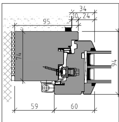
Schnitt seitlich
