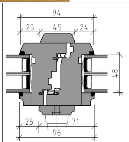
Schnitt Mittelpartie
