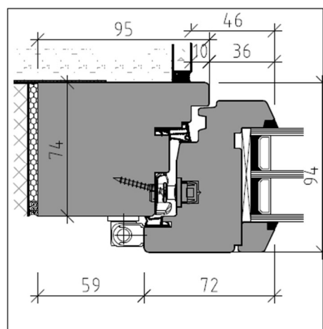
Schnitt seitlich
