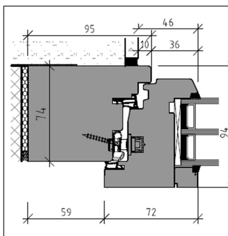
Schnitt seitlich
